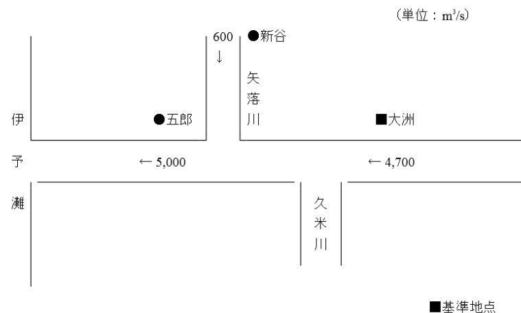
図-3 肱川計画高水流量図
