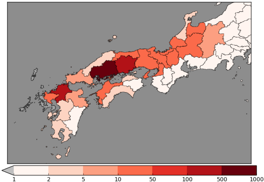
県平均最大24時間雨量の再起年数
